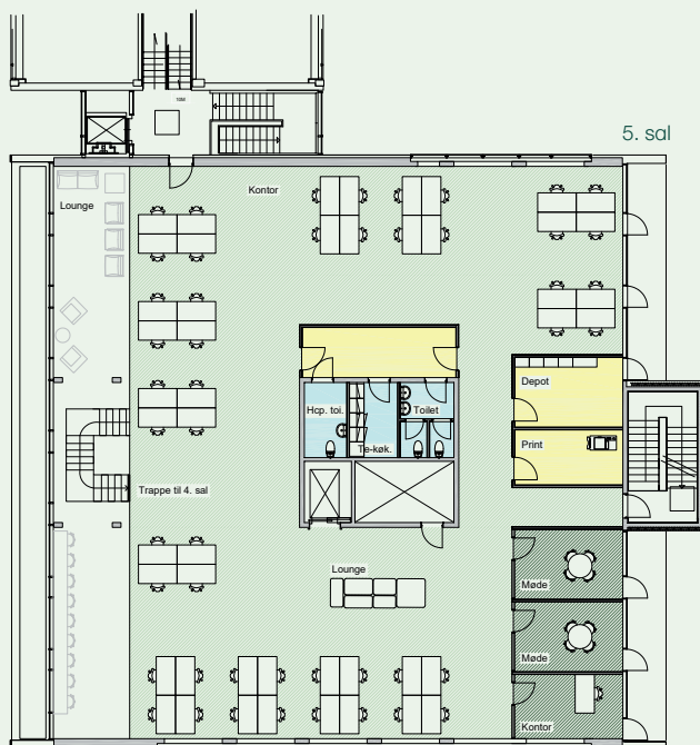
Vejledende indretningsforslag
